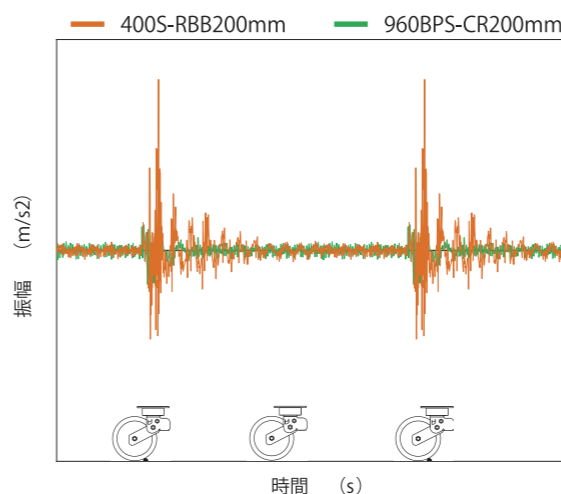
時間軸波形
